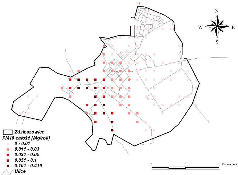
Rysunek 65 Całkowita emisja liniowa pyłu zawieszonego PM 10 w Zdieszowicach w 2006 r.
