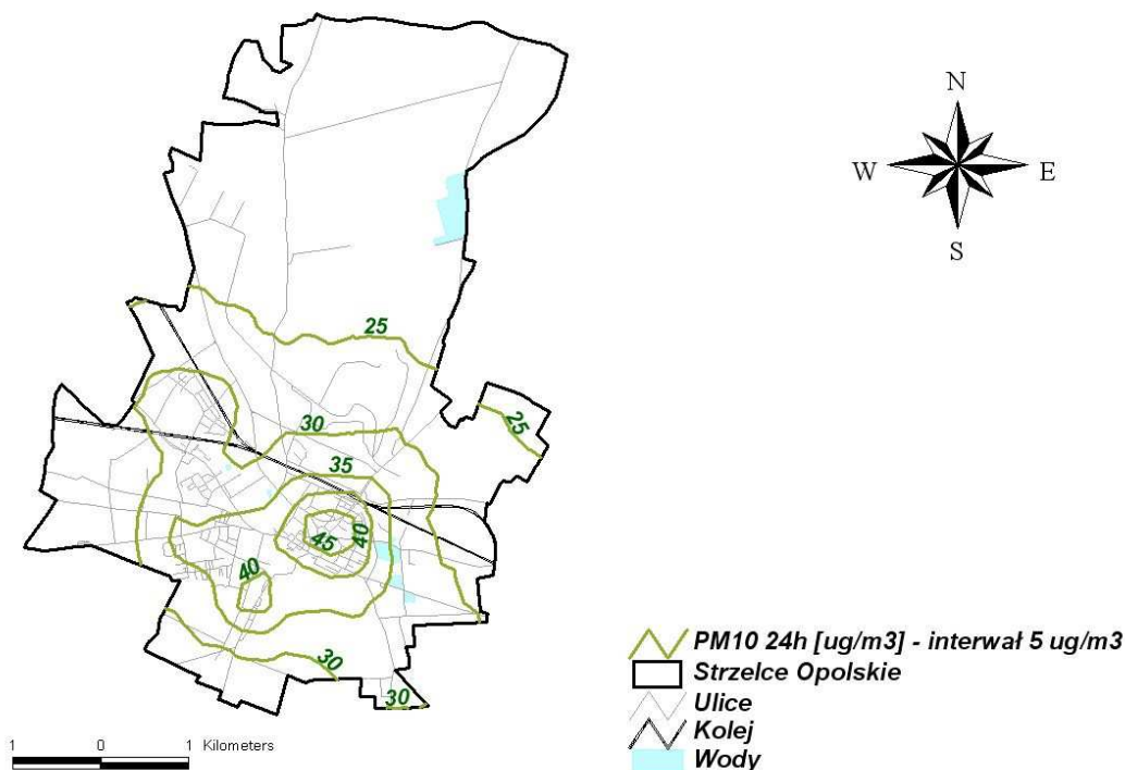
Rysunek 168 Rozkład stężeń pyłu zawieszonego PM_{10} o okresie uśredniania wyników pomiarów 24 godziny pochodzących od całkowitej emisji, po zastosowaniu wariantu komunikacyjnego, powierzchniowego oraz obniżeniu emisji napływowej na teren Strzelce Opolskich
