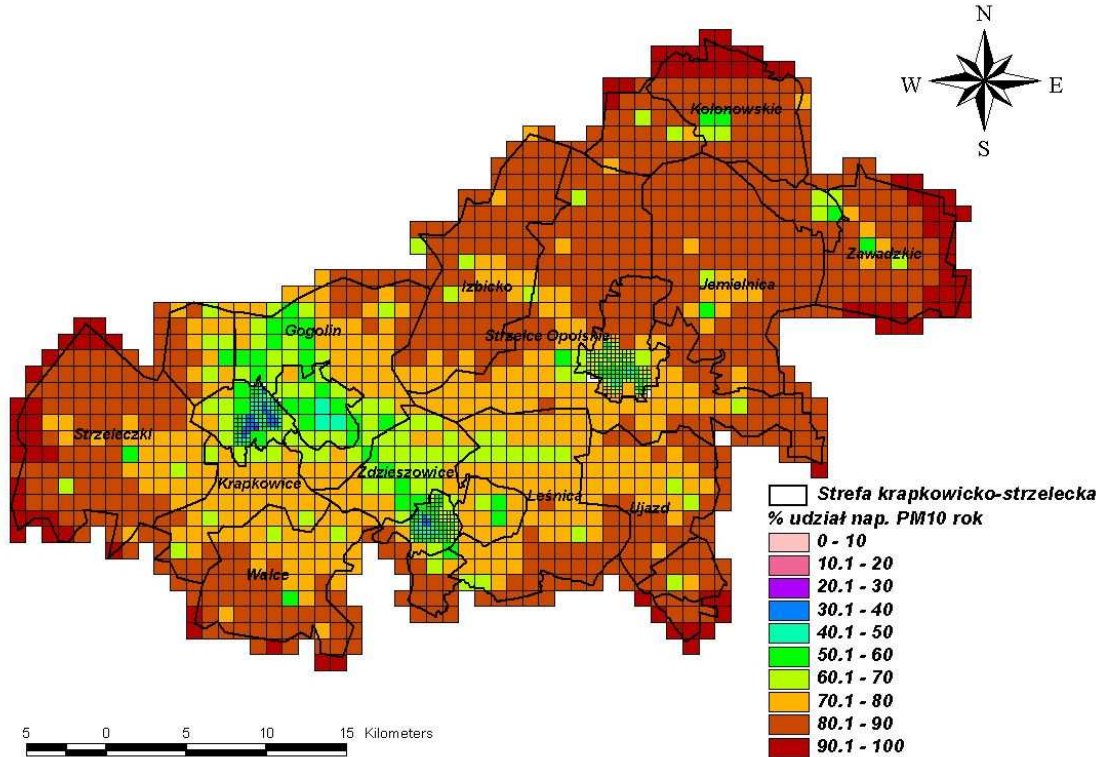
Rysunek 137 Procentowy udział emisji napywowej w stężeniach pyłu zawieszonego PM_{10} o okresie uśredniania wyników pomiarów rok kalendarzowy na terenie strefy krapkowicko-strzeleckiej w 2006 r.
