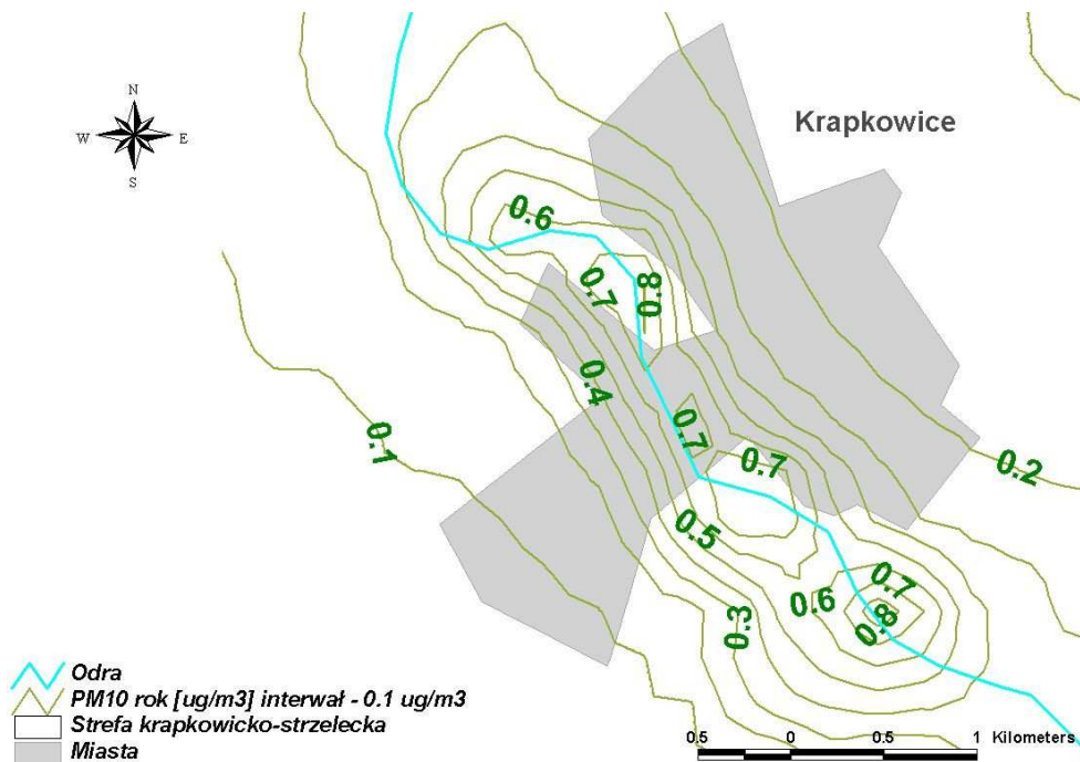
Rysunek 123 Rozkład stężeń pyłu zawieszonego PM10 o okresie uśredniania wyników pomiarów rok kalendarzowy pochodzących od emisji z transportu Odrą w Zdziechowicach w 2006 r.
