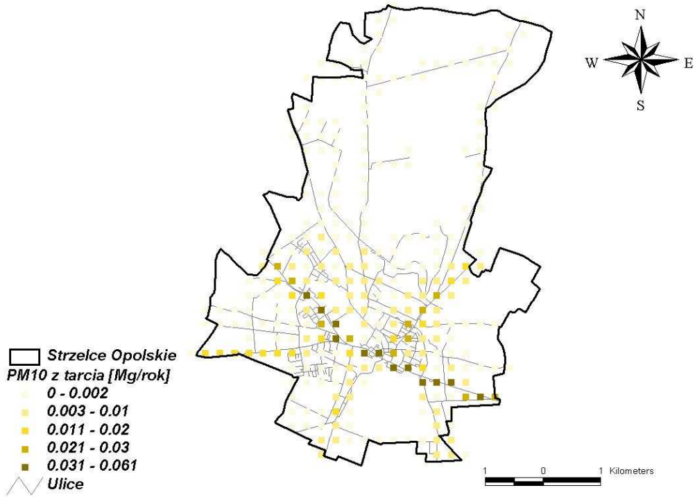
Rysunek 64 Emisja pyłu zawieszonego PM 10 z tarcia, ze źródeł komunikacyjnych w Strzelcach Opolskich w 2006 r.
